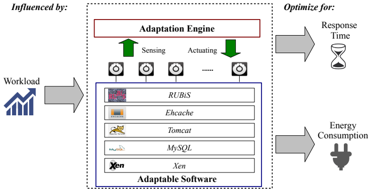
Fig. 1. An example of SAS.
